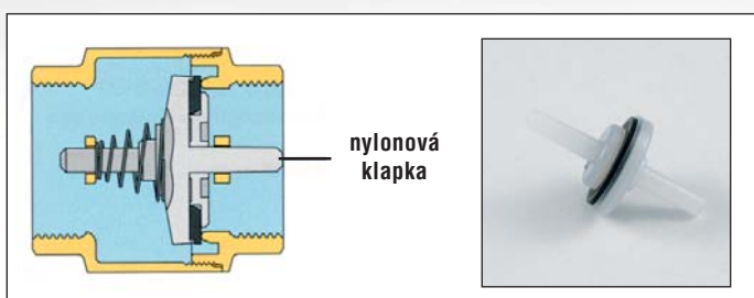
Art. TM 3660 vodorovná zpětná klapka FULL ISO 228, T = -20° - 110°C
