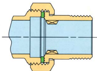
Řez artiklem "CP" - radiátorové šroubení těsnící na plocho
